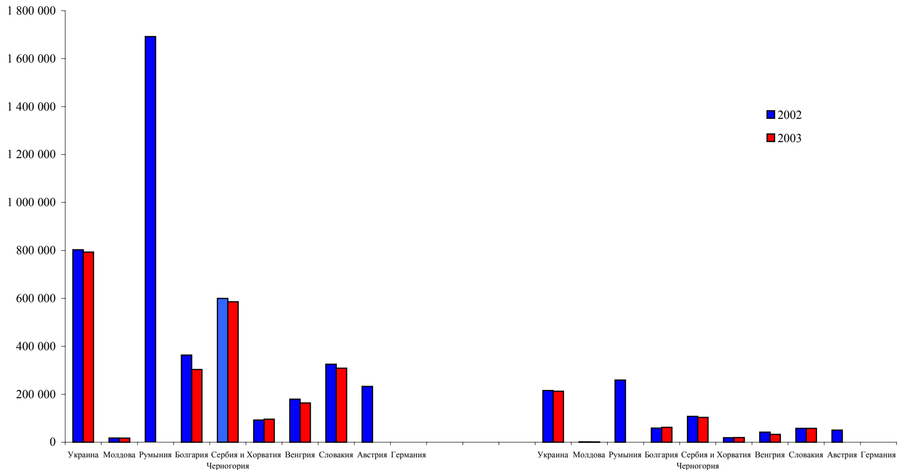
Рис. П.2 РАЗВИТИЕ ГРУЗОПОДЪЕМНОСТИ ДУНАЙСКОГО ФЛОТА В ПРИДУНАЙСКИХ СТРАНАХ В 2003 ГОДУ ПО СРАВНЕНИЮ С 2002 ГОДОМ (тыс. т)
