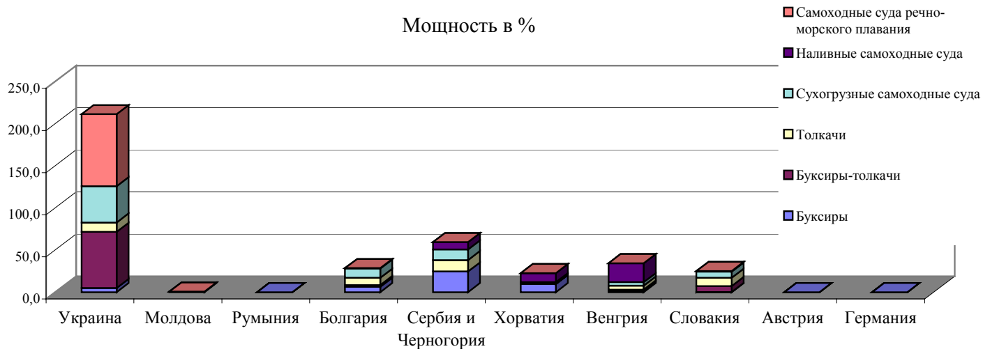
Рис. П.4 НАЛИЧИЕ ФЛОТА НА ДУНАЕ С РАЗБИВКОЙ ПО ТИПАМ СУДОВ, КАТЕГОРИЯМ ГРУЗОПОДЪЕМНОСТИ И МОЩНОСТИ
