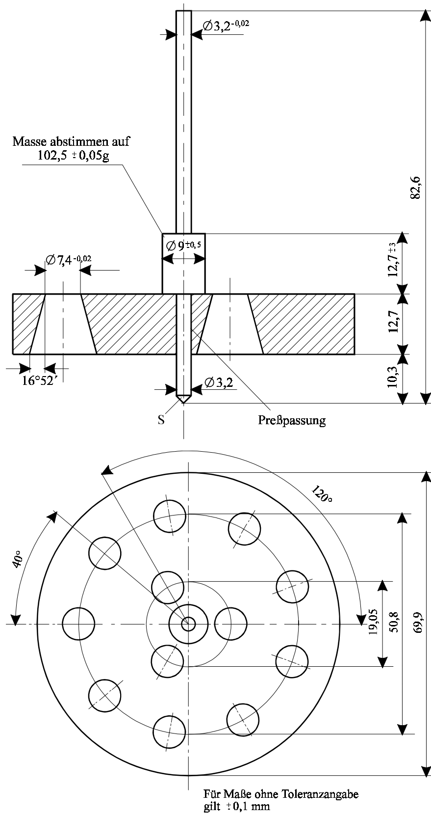
Abbildung 4 Penetrometer
