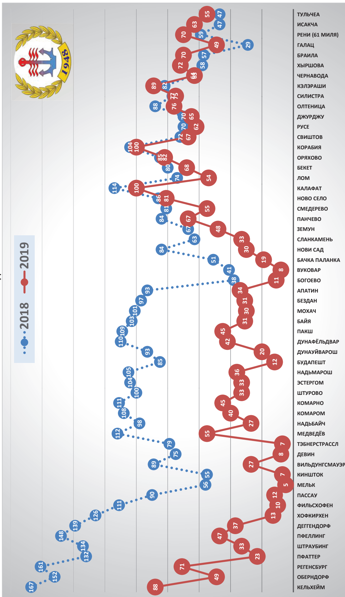
I.D. Количество дней с уровнями воды ниже значения НСРУ на некоторых водомерных постах на судоходном участке реки Дунай в течение года
